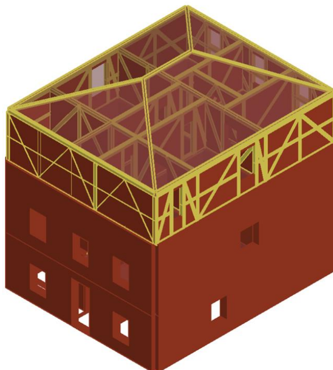
Slika 61 3D model zgrade - jugozapadna strana
