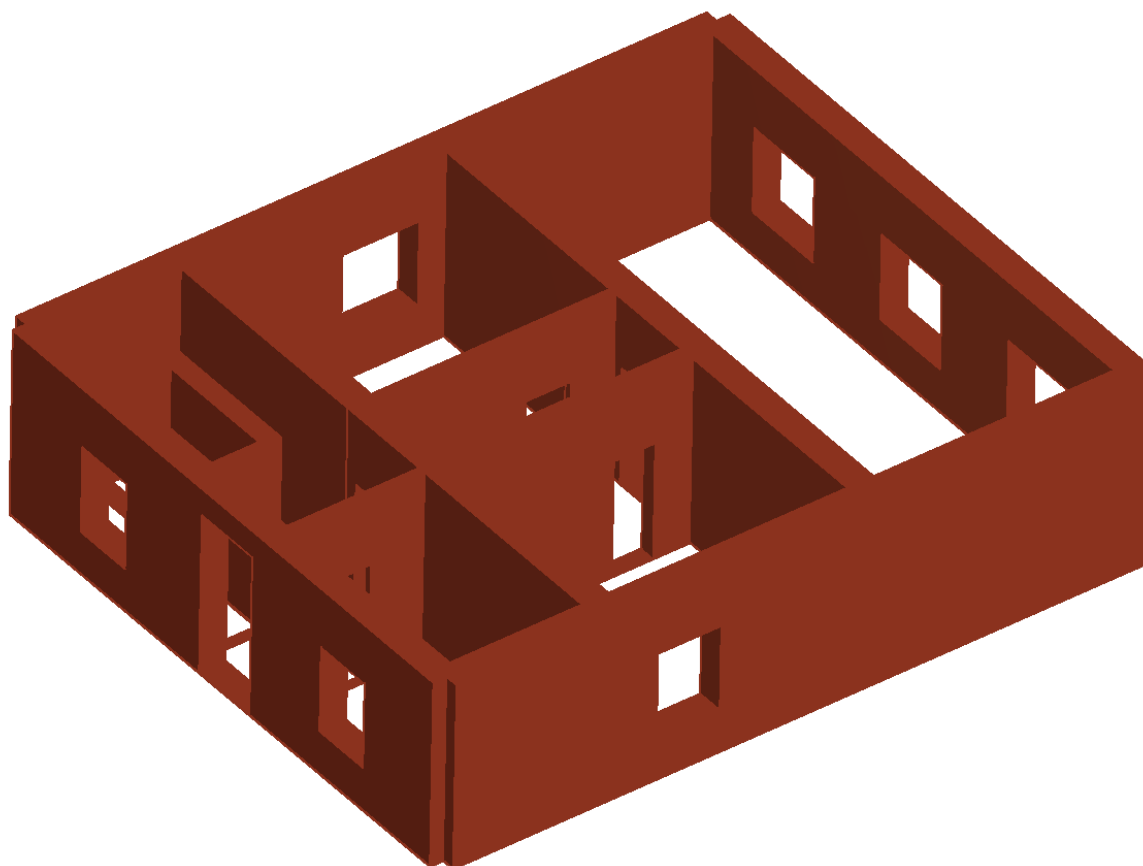
Slika 92 3D prikaz prizemlja modela
