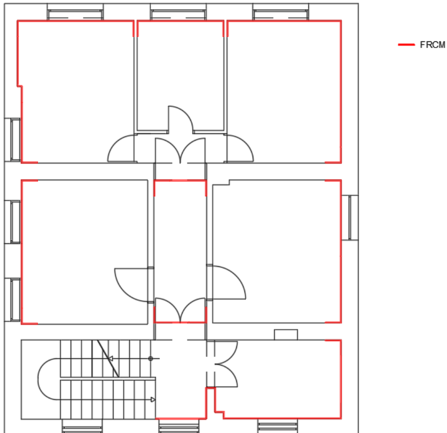
Slika 77: 1. kat – lokacije FRCM sustava za ojačanje zidova
