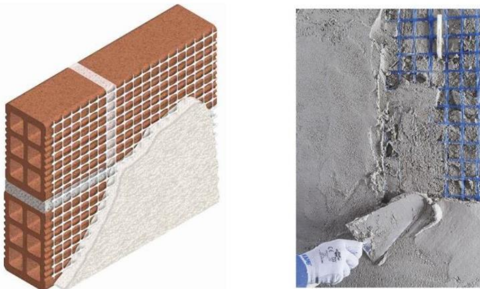
Slika 71 Detalji izvedbe ojačanja FRCM sustavom
