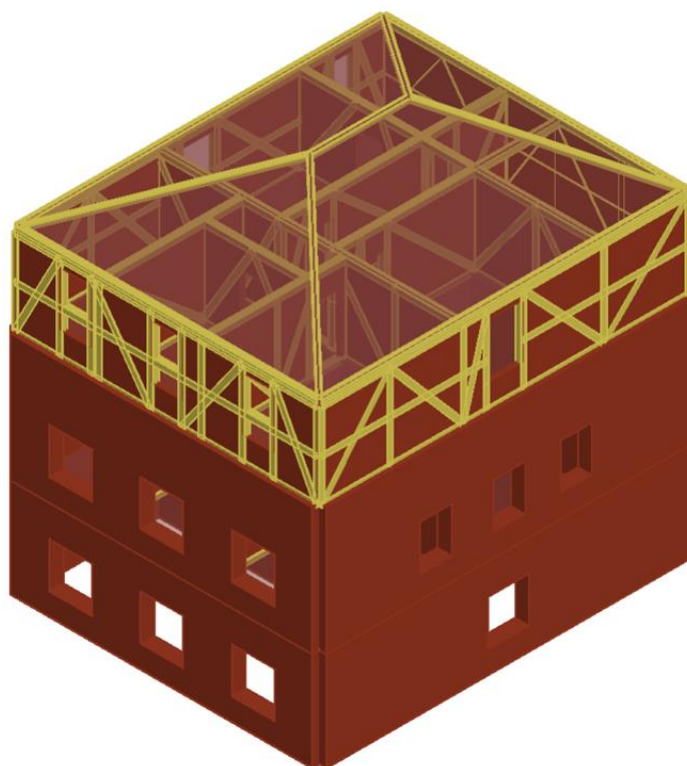
Slika 95 3D model zgrade - sjeveroistočna strana
