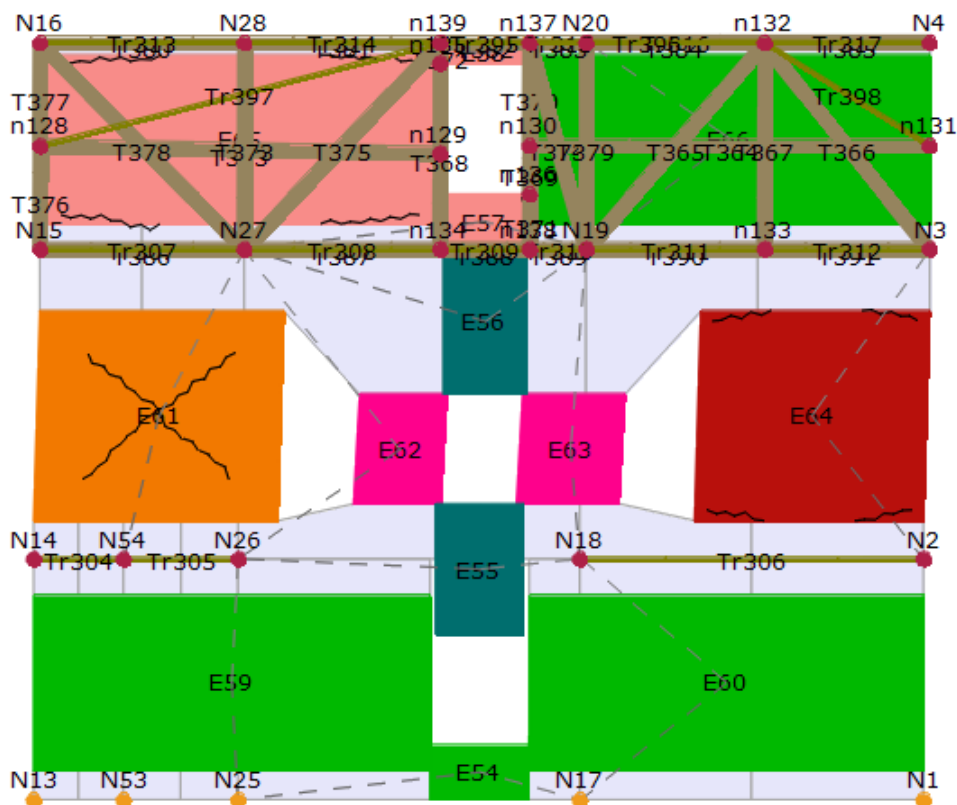
Slika 66 Prikaz deformacija zida sjevernog pročelja (zid P4)
