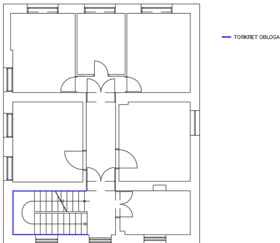
Slika 82: 1. kat – lokacije torkret obloge za ojačanje zidova
