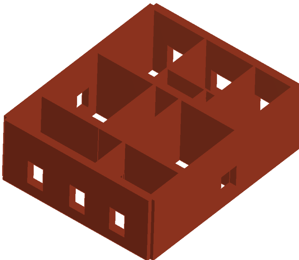
Slika 58 3D prikaz 1. kata modela
