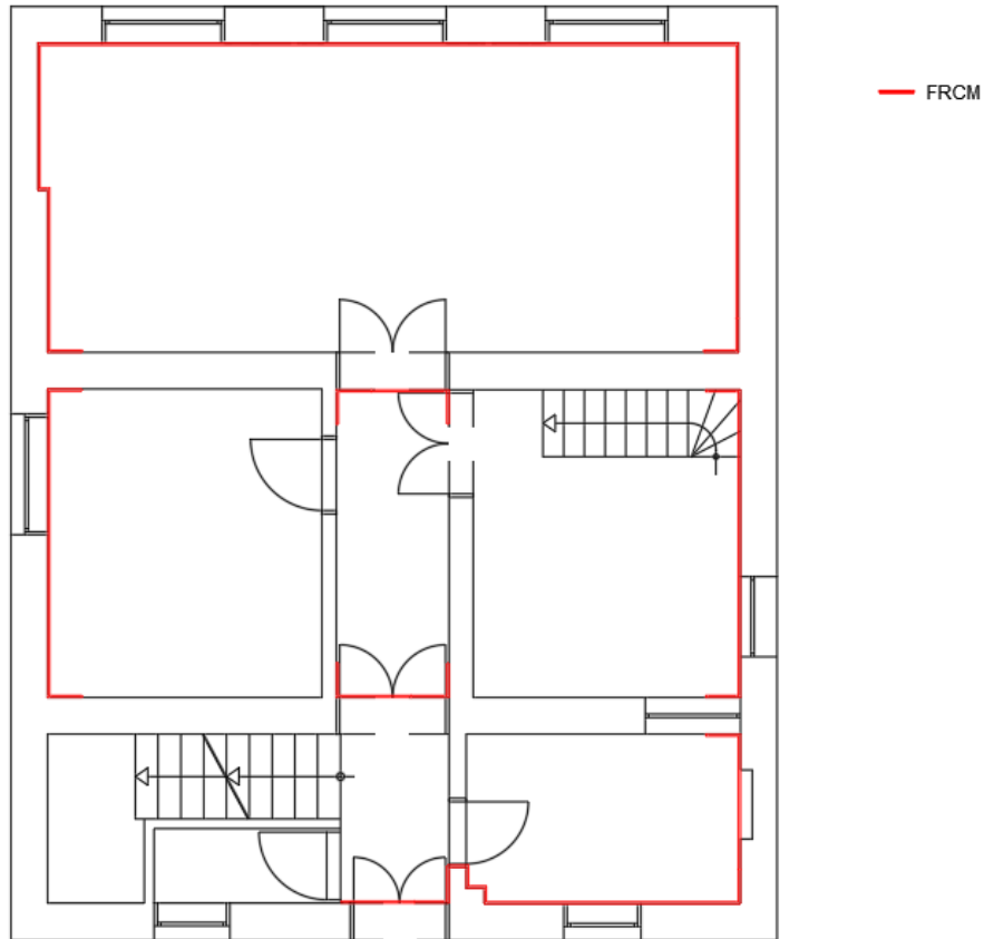
Slika 76: Prizemlje – lokacije FRCM sustava za ojačanje zidova
