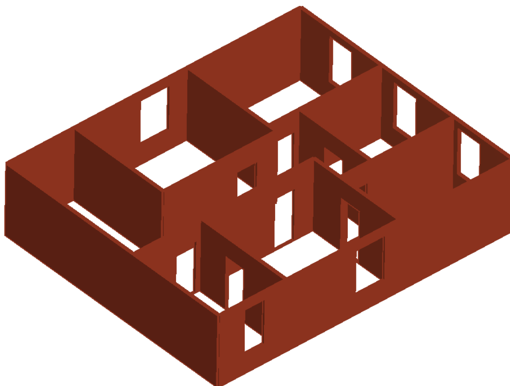
Slika 59 3D prikaz potkrovlja modela
