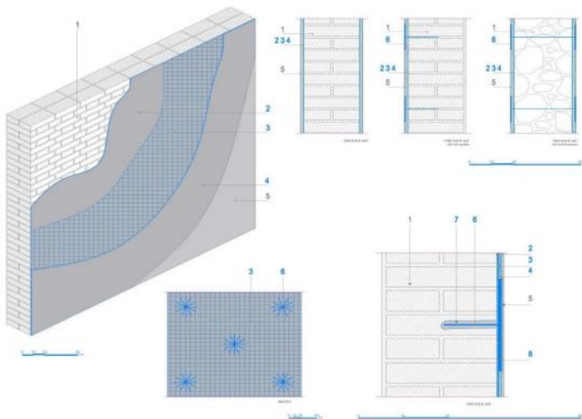
Slika 73 Detalji izvedbe ojačanja FRCM sustavom - redoslijed izvođenja sustava
