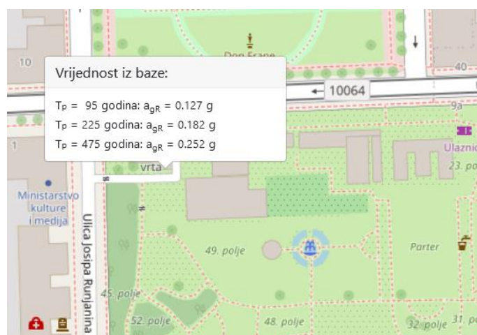
Slika 98: Prikaz vršnih ubrzanja tla za lokaciju - Karte potresnih područja Republike Hrvatske
