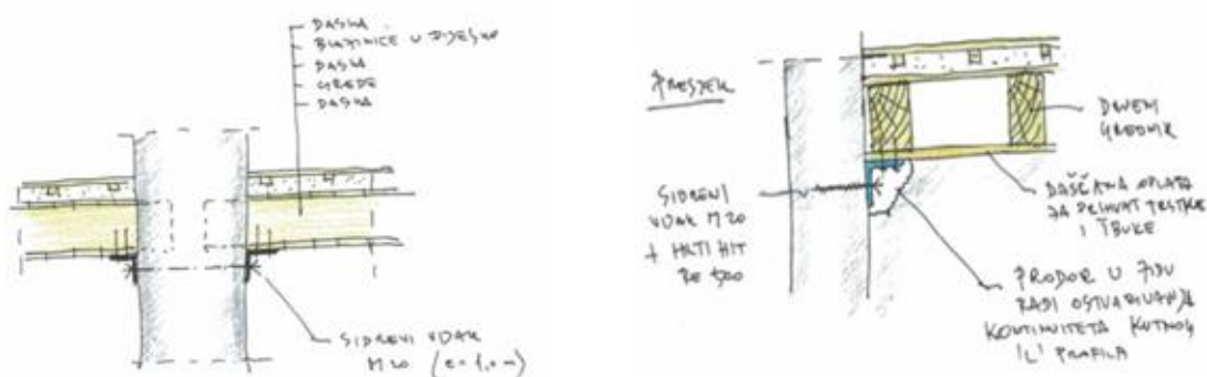
Slika 84: Detalji spajanja sa zidom
