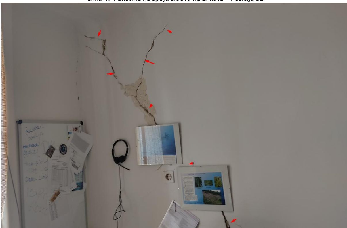
Slika 48 Pukotine na zidu na 2. katu – Pozicija 33
