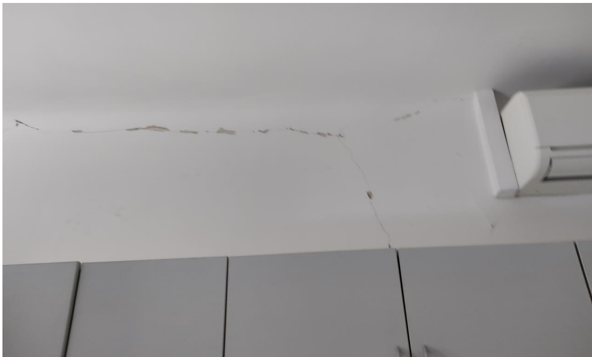
Slika 45 Pukotine na spoju zida sa stropnom konstrukcijom na 2. katu – Pozicija 30
