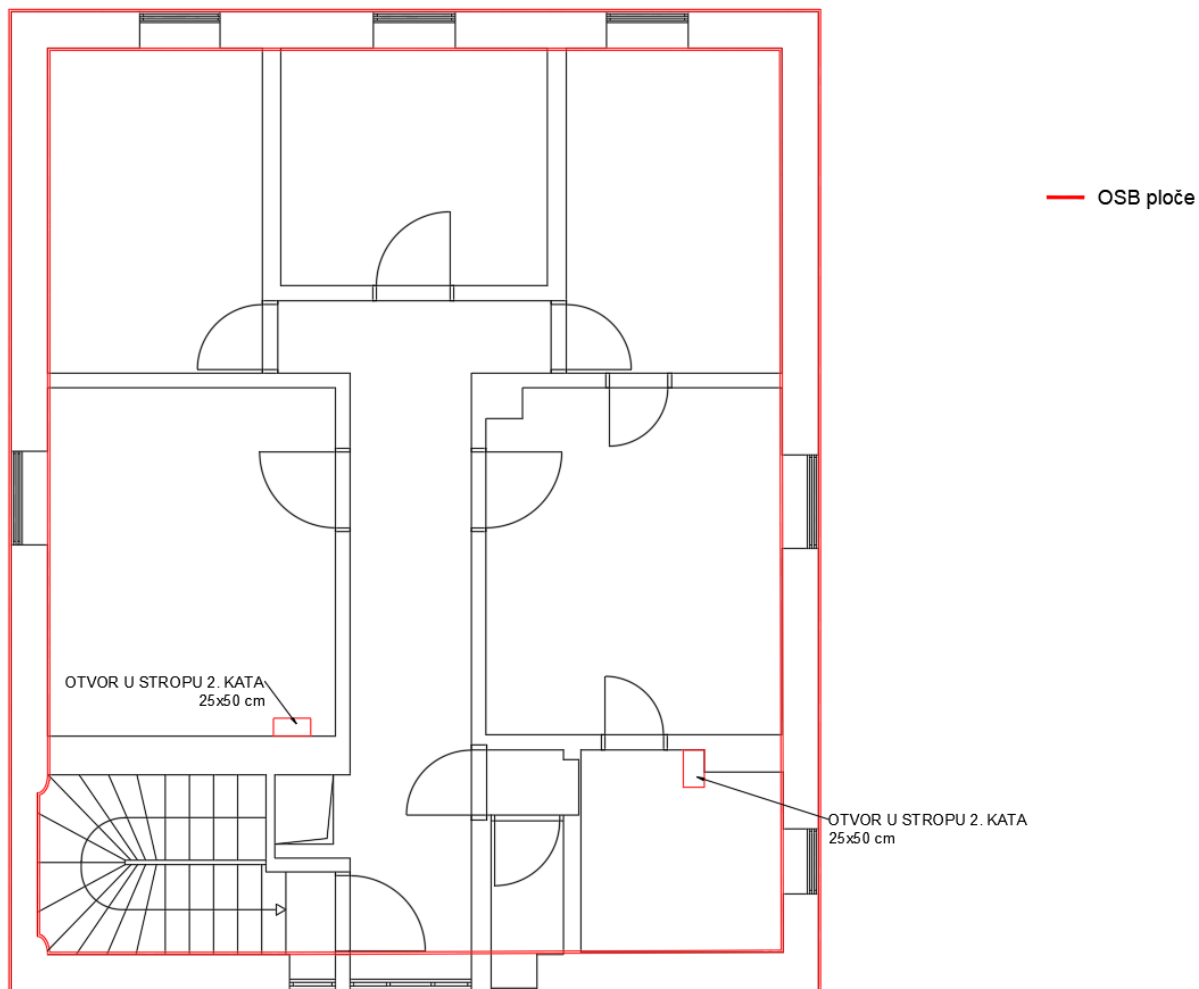
Slika 87: Potkrovlje - lokacije ojačanja mansardnog dijela krovništva OSB pločama
