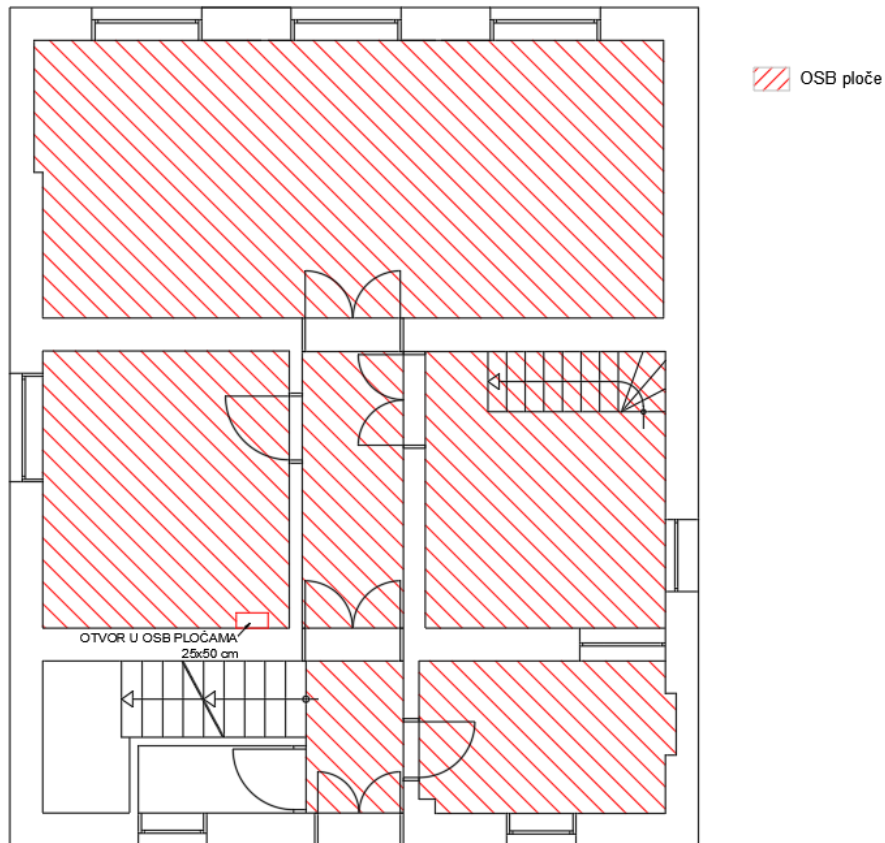
Slika 85: Prizemlje - lokacije ojačanja međukatne konstrukcije OSB pločama
