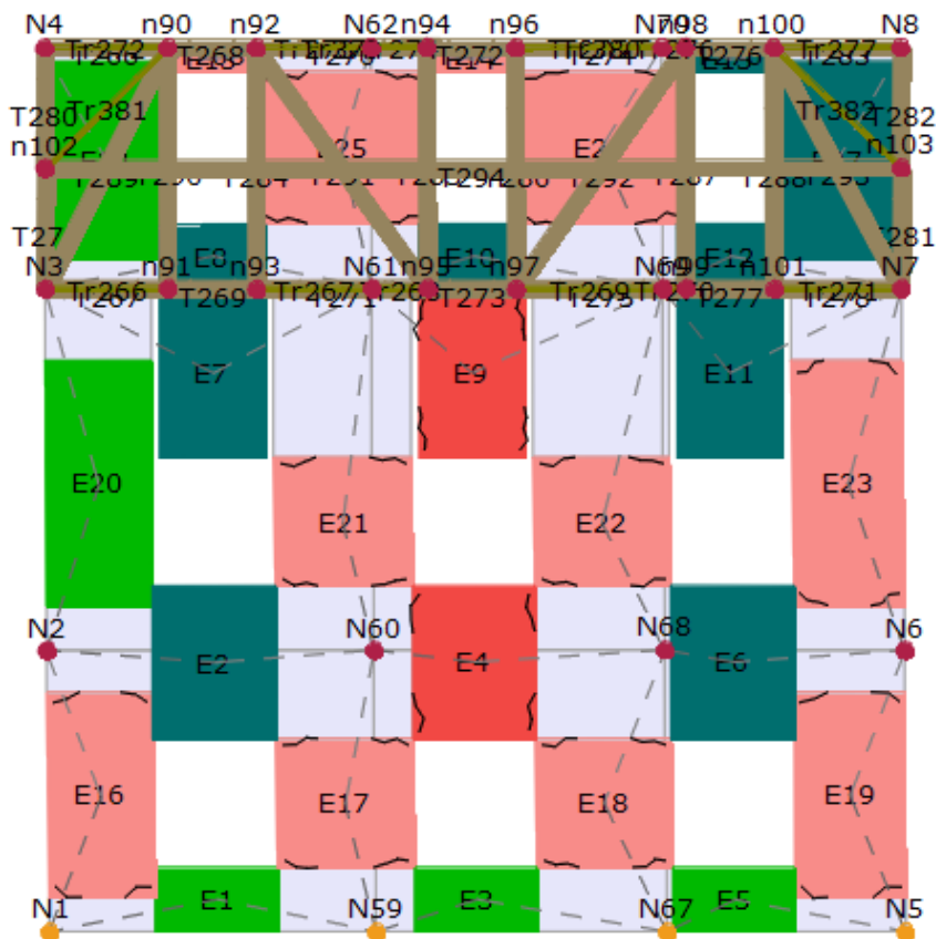
Slika 64 Prikaz deformacija zida istočnog pročelja (zid P1)
