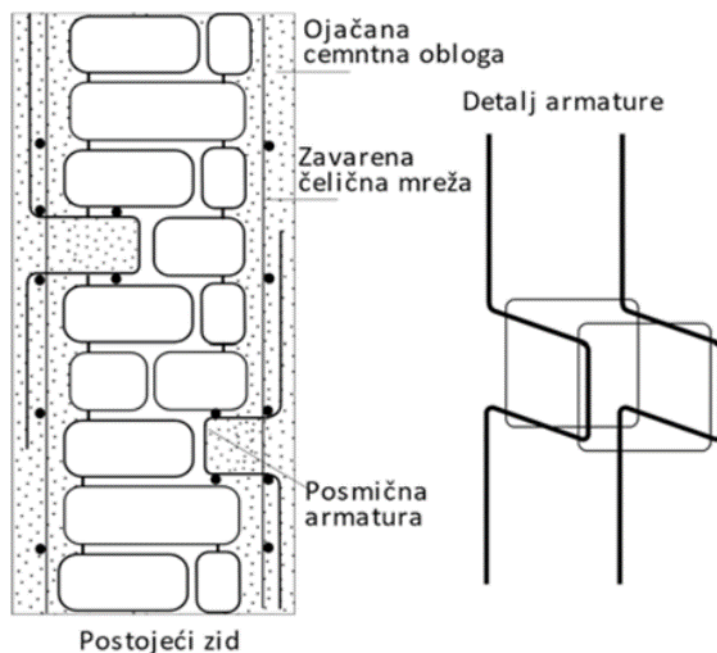
Slika 78: Grafički prikaz postavljanja armiranobetonske obloge
