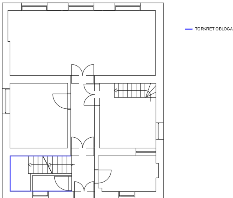
Slika 81: Prizemlje – lokacija torkret obloge za ojačanje zidova
