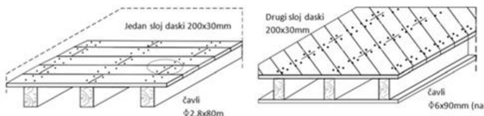
Slika 83: Postavljanje OSB ploča ispod grednika
