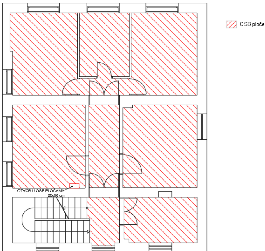
Slika 86: 1. kat - lokacije ojačanja međukatne konstrukcije OSB pločama
