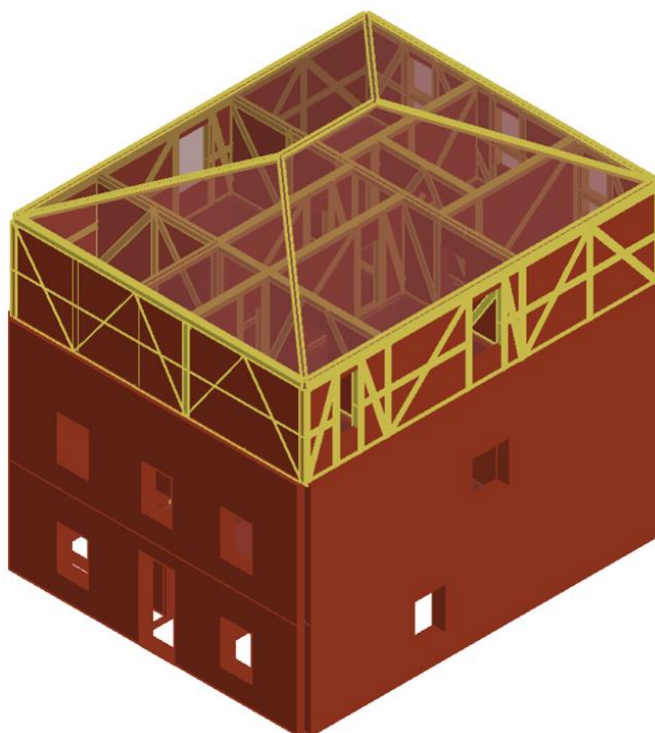
Slika 96 3D model zgrade - jugozapadna strana
