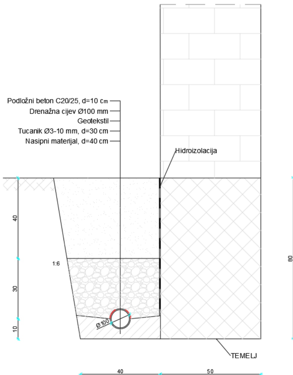
Slika 91: Prikaz izvedbe drenažnog sustava
