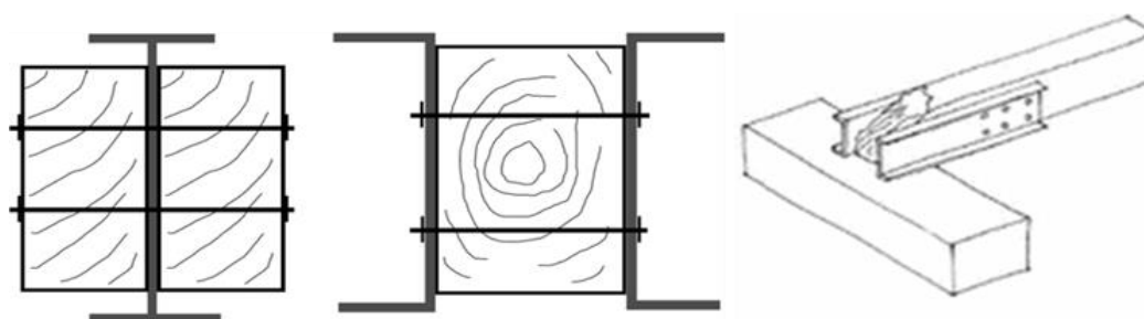
Slika 89: Sanacija i pojačanje drvenih elemenata dodavanjem čeličnih elemenata
