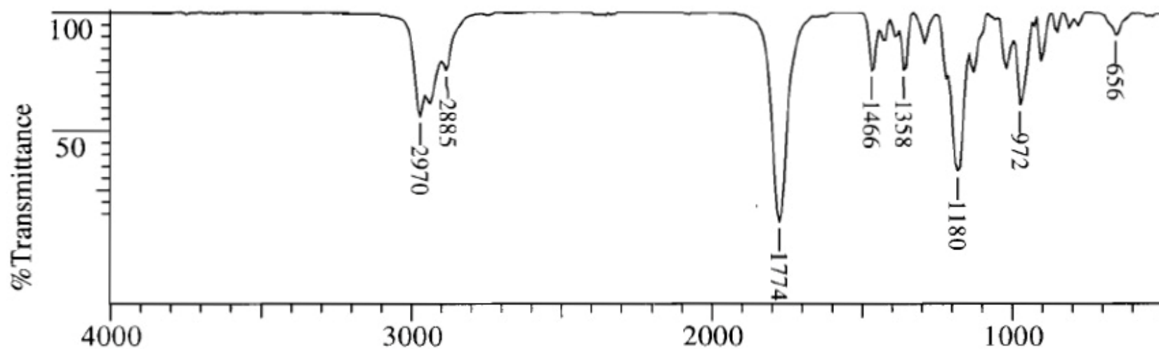
IR spektar
