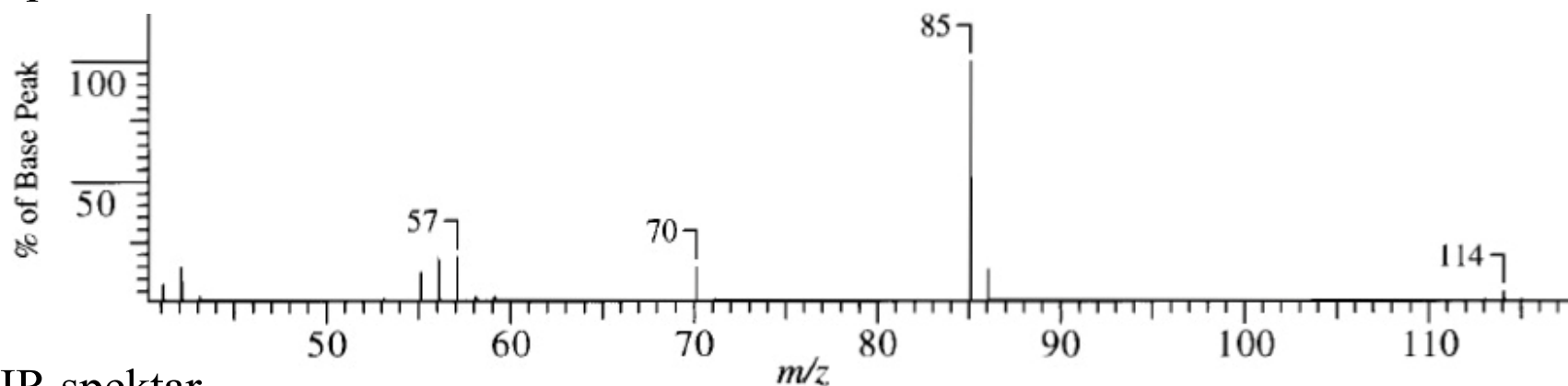
Spektar MS
