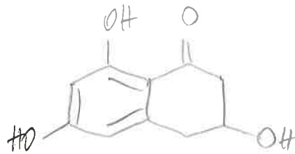
skitalon poliketid
