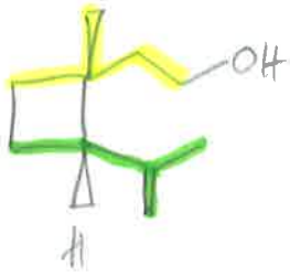
grandisol monoterpen
